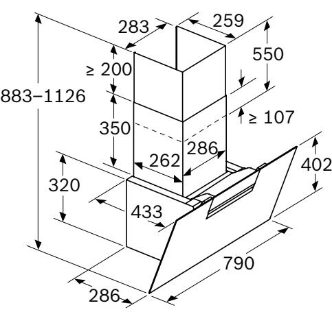
Aparato en salida de aire al exterior
