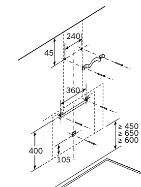
Instalación en pared con conducto
