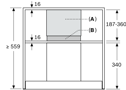
Ejemplo de montaje para altura de armario ≥559 mm
