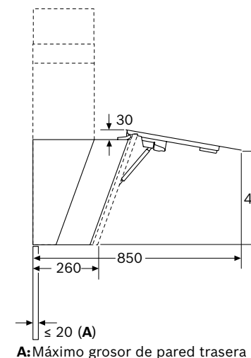
Instalación en pared con conducto
