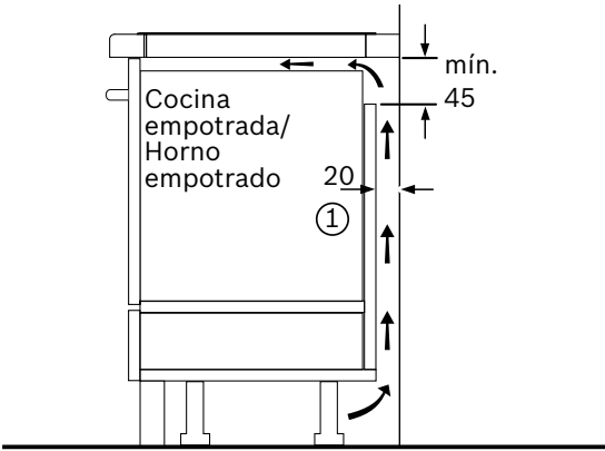
① Rendija de ventilación necesaria
