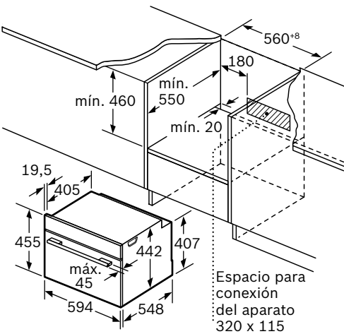
Montaje con una placa
