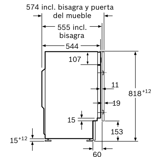
Detalle Z
