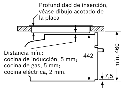
Montaje con una placa
