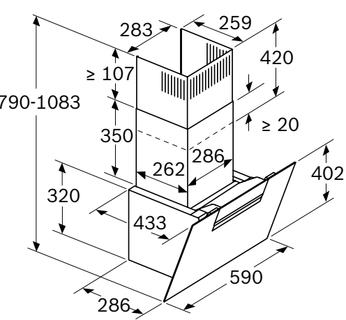
Aparato en recirculación
