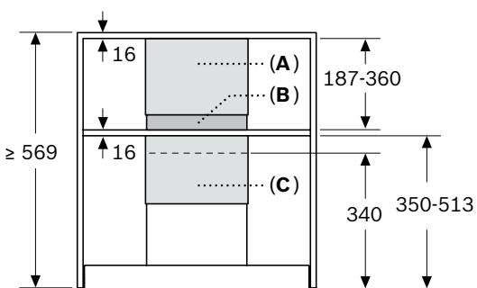
Ejemplo de montaje para altura de armario ≥569 mm
