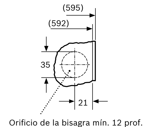
Detalle Z
