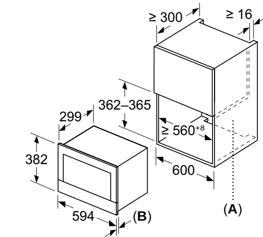
A: Pared trasera abierta B: 19,5 mm
