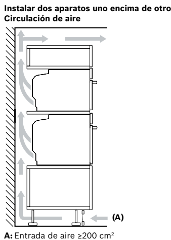
A: Entrada de aire ≥200 cm²
