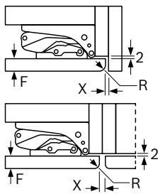
Dimensiones del espacio recomendadas para instalación de puerta fija
