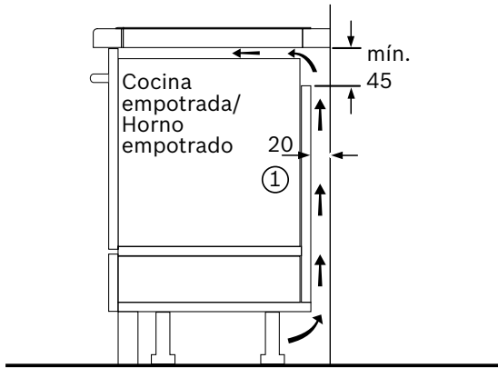
① Rendija de ventilación necesaria
