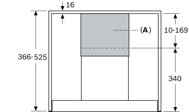
Ejemplo de montaje para altura de armario de 366-525 mm
