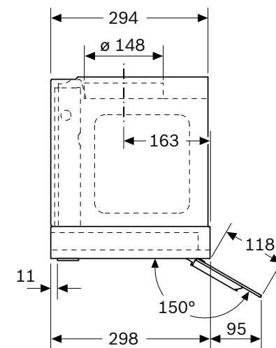
Vista lateral
