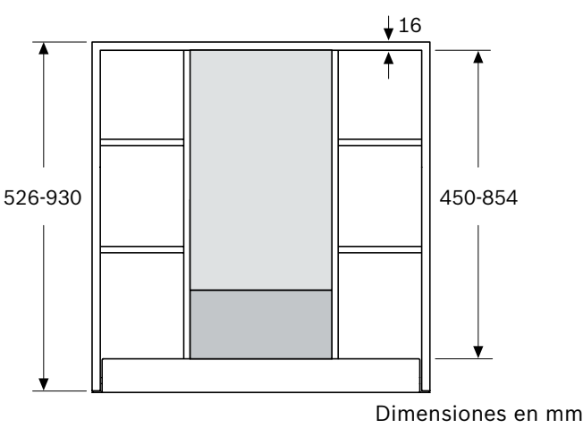
Ejemplo de montaje para altura de armario de 526-930 mm con estantes laterales
