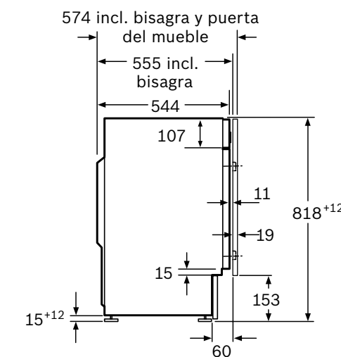
Detalle Z
