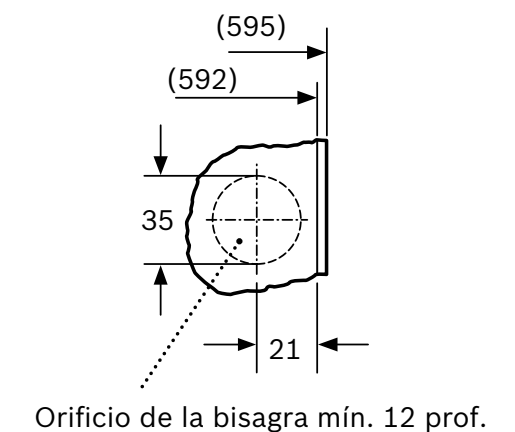
Detalle Z
