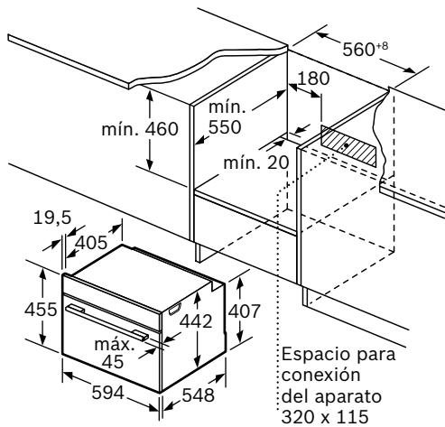
Montaje con una placa
