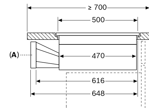
A: Adaptador cilíndrico/plano
