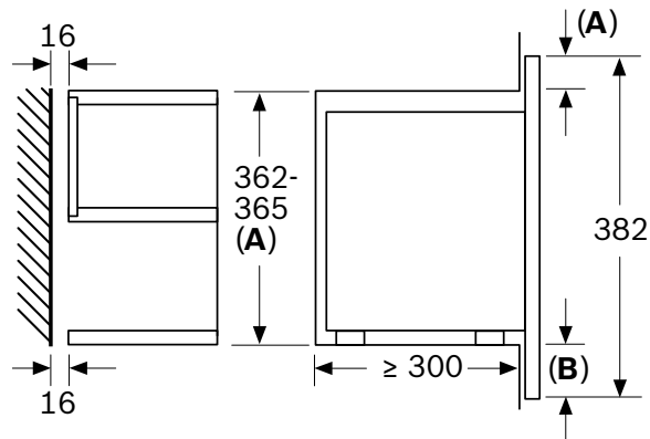
A: Saliente superior: Hueco 362: 6 mm Hueco 365: 3 mm B: Saliente inferior: 14 mm
